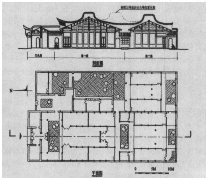
图4 陈承裘故居平面与剖面图
