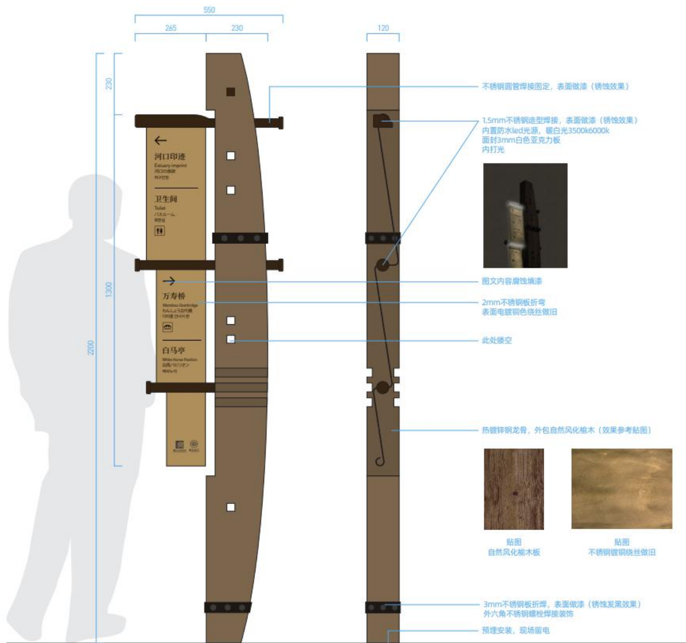
正视图 1:10
