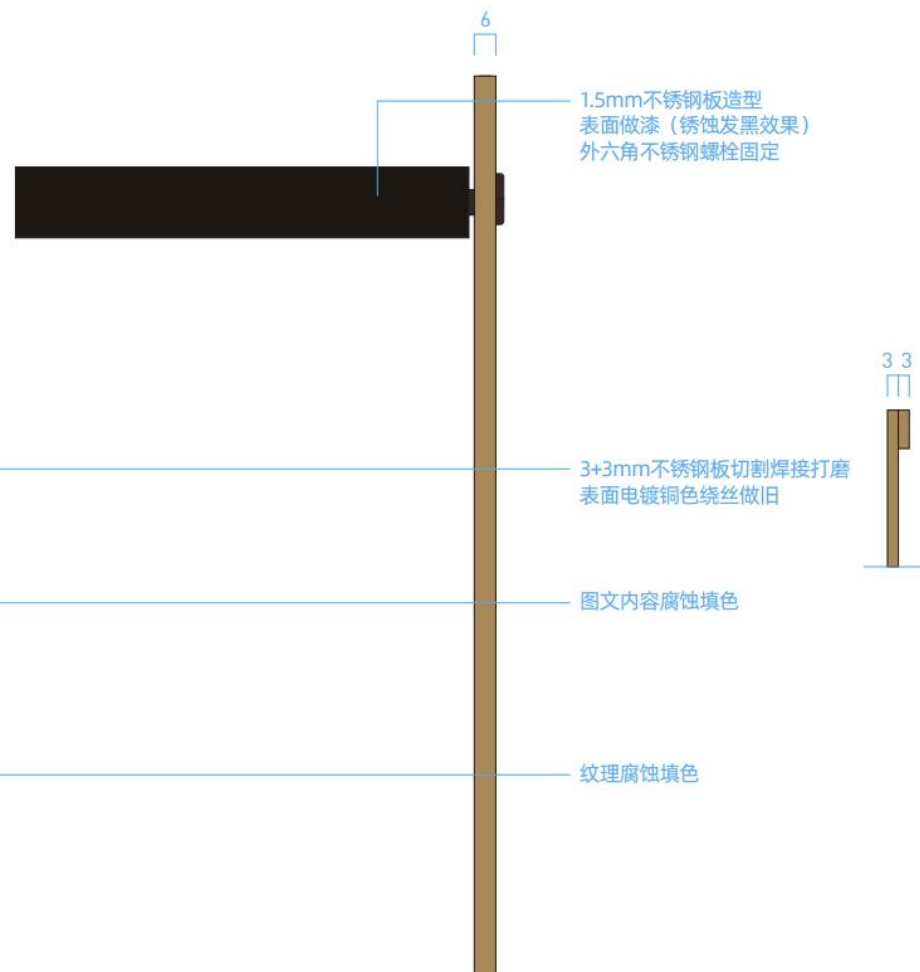
侧视图 1:2
