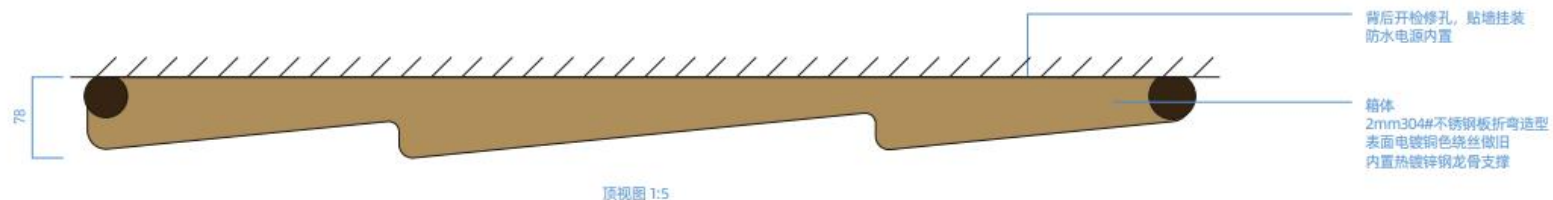
顶视图 1:5
